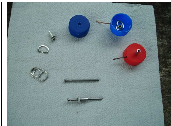
Figura 6 – detalhes adicionais da “flor” anti-abelha
